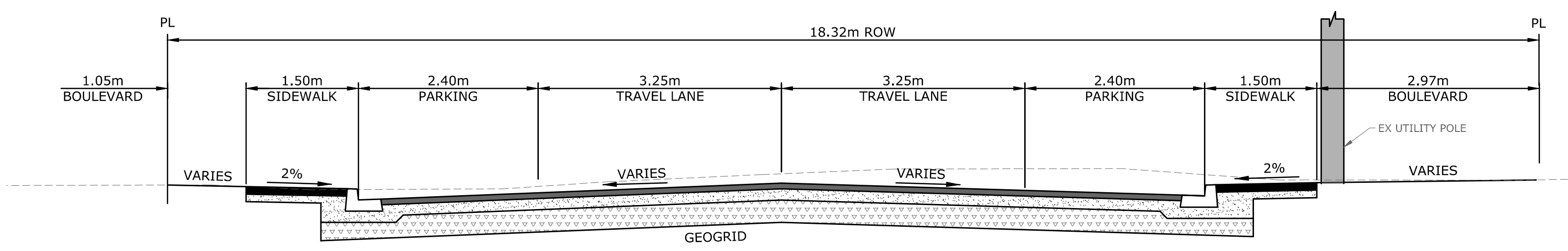
A-A TYPICAL ROAD SECTION - OPTION A SCALE: N.T.S.
