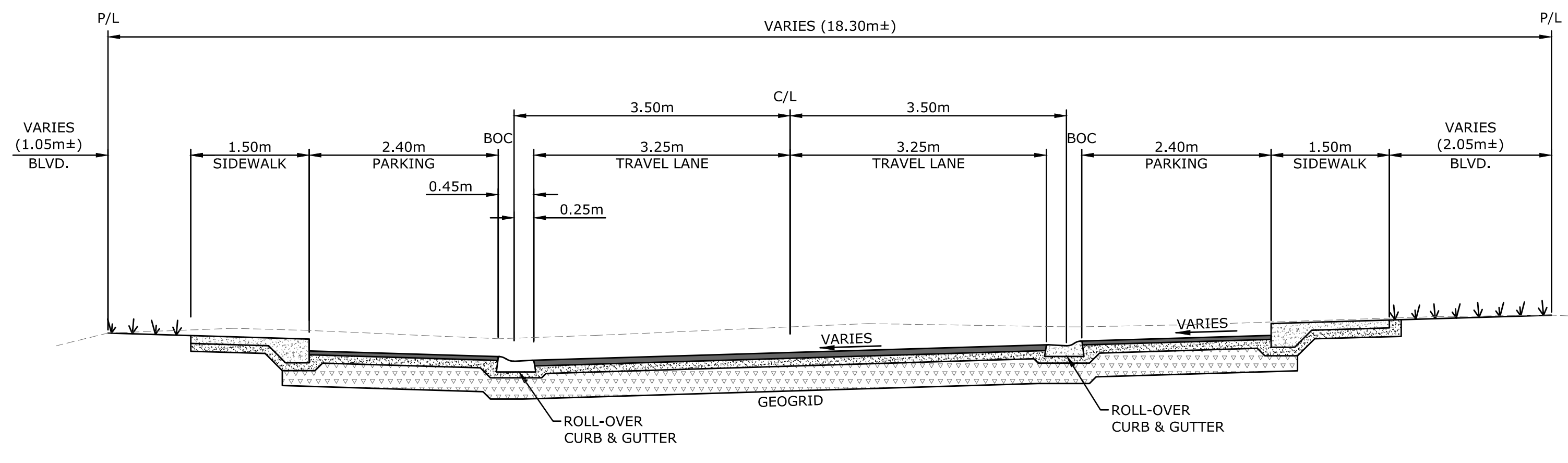
D-D TYPICAL ROAD SECTION - OPTION B SCALE: N.T.S
