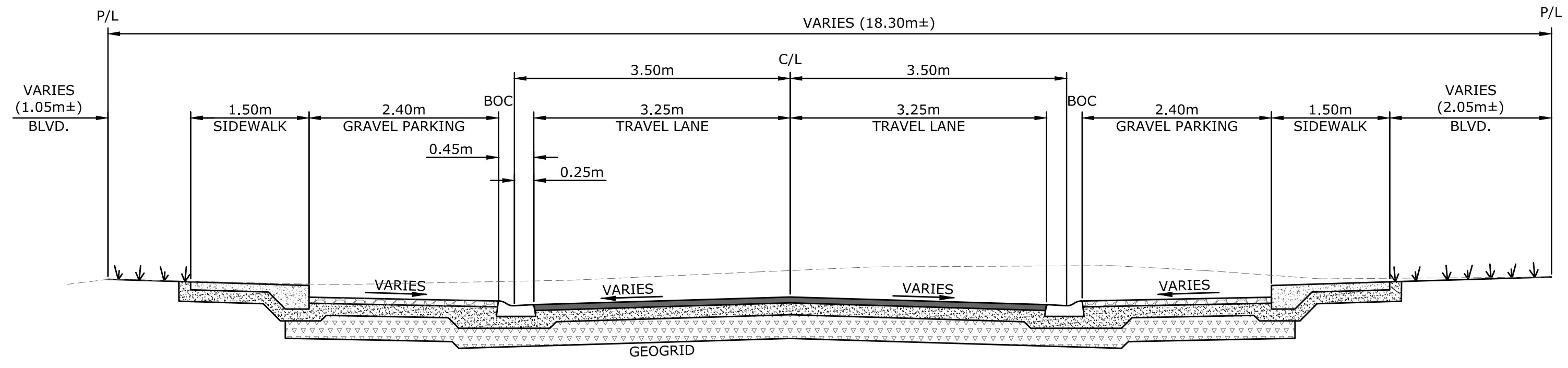
C-C TYPICAL ROAD SECTION - OPTION B SCALE: N.T.S
