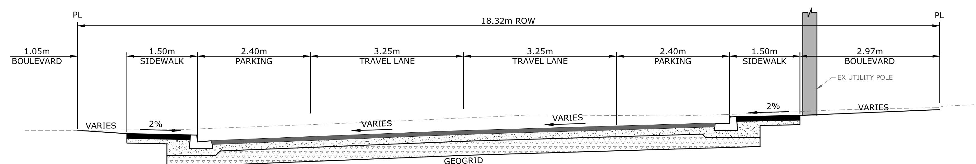
B-B TYPICAL ROAD SECTION - OPTION A SCALE: N.T.S.
